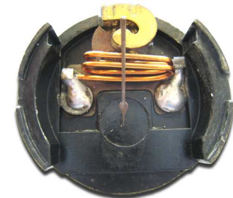
Revidiertes Amperemeter
