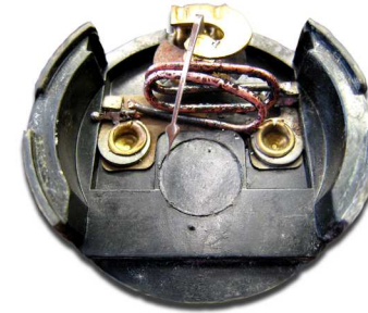
Verbranntes Amperemeter
